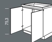
SP_H Spülen-Unter- schrank Base unit for sink Breite Width 80, 90, 100 cm
