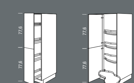
SA_V Seitenschrank für Vorräte Tall unit for food storage Breite Width 30, 45 cm
