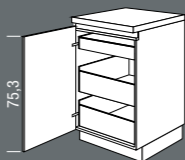
UISIA_H Unterschrank Base unit Breite Width 30, 45, 50, 60 cm
