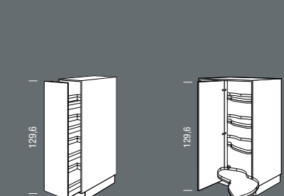
SA_V Seitenschrank für Vorräte Tall unit for food storage Breite Width 30, 45 cm
