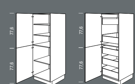
S_V Seitenschrank Tall unit Breite Width 30, 45, 50, 60 cm
