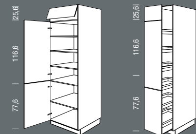
S_V Seitenschrank Tall unit Breite Width 30, 45, 50, 60 cm
