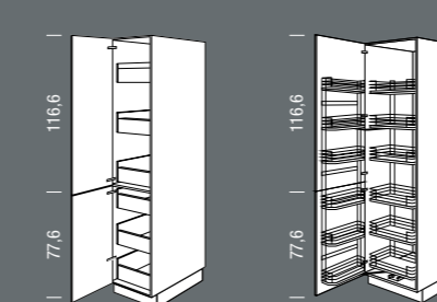
SIA_V Seitenschrank für Vorräte Tall unit for food storage Breite Width 30, 45, 50, 60 cm
