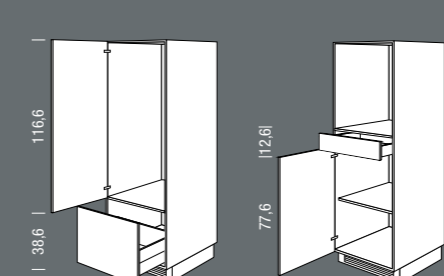
SU_V Seitenschrank für Kühlgerät Tall unit for refrigerator Breite Width 60 cm
