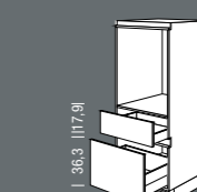
SUBSA_H Seiten- schränk für Backofen Tall unit for oven Breite Width 60 cm
