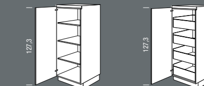
S_H Seitenschränk Tall unit Breite Width 30, 45, 50, 60 cm SIA_H Seitenschränk Tall unit Breite Width 30, 45, 50, 60 cm
