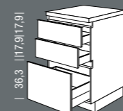
U2SA_H Unterschrank Base unit Breite Width 30, 40, 45, 50, 60, 80, 90, 100, 120 cm
