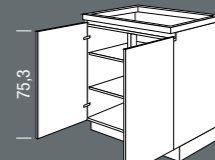
U_H Unterschrank Base unit Breite Width 80, 90, 100 cm
