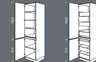
S_H Seitenschränk Tall unit Breite Width 30, 45, 50, 60 cm SIA_H Seitenschränk Tall unit Breite Width 30, 45, 50, 60 cm
