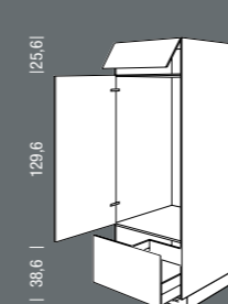
SU_V Seitenschrank für Kühlgerät Tall unit for refrigerator Breite Width 60 cm
