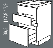
UKSA_H Unterschrank mit Kochmulde Base unit with hob Breite Width 60, 90 cm
