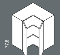
HE_H Eck-Hänge- schrank Corner wall unit Breite Width 60, 65 cm
