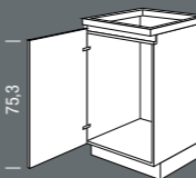
SP_H Spülen-Unter- schrank Base unit for sink Breite Width 45, 50, 60 cm
