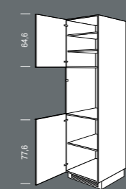
SUB_V Seitenschrank für Backofen Tall unit for oven Breite Width 60 cm
