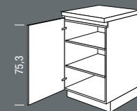
U_H Unterschrank Base unit Breite Width 30, 40, 45, 50, 60 cm
