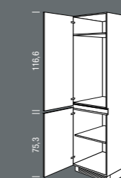
SU_H Seitenschränk für Kühlgerät Tall unit for refrigerator Breite Width 60 cm
