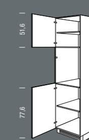
SUB_V Seitenschrank für Backofen Tall unit for oven Breite Width 60 cm
