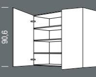
H_H Hängeschränk Wall unit Breite Width 80, 90, 100 cm
